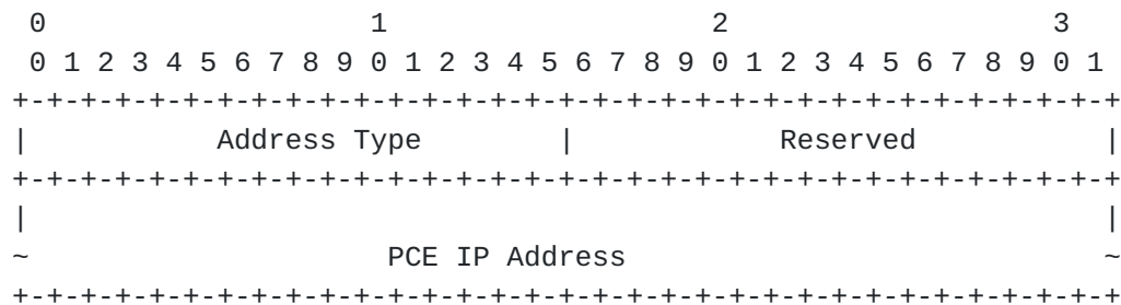
PCE-ID TLV format
