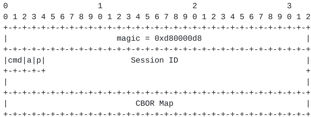
Figure 2: SPUD packets
