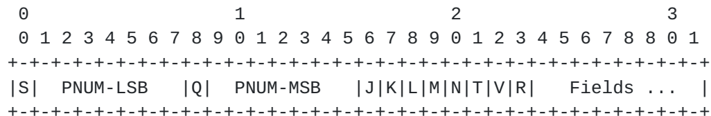
Figure A.4.2 -- Parameter log format
