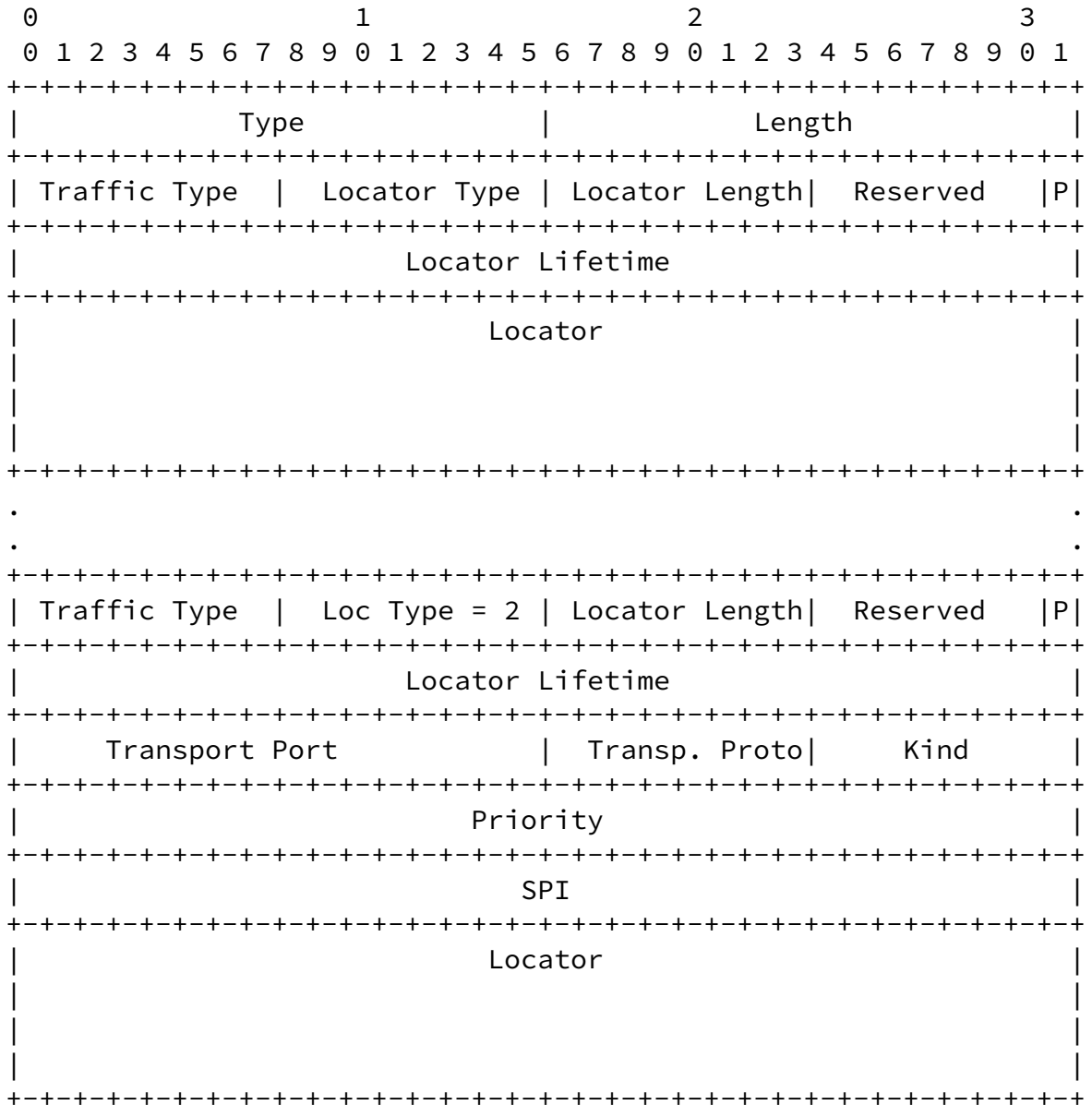
Figure 9: LOCATOR parameter
