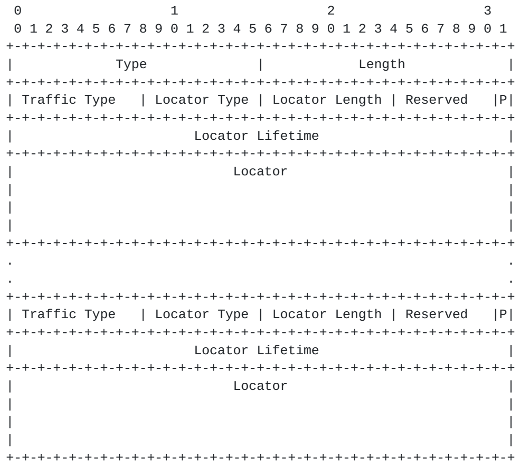
Figure 12: LOCATOR Parameter Format
