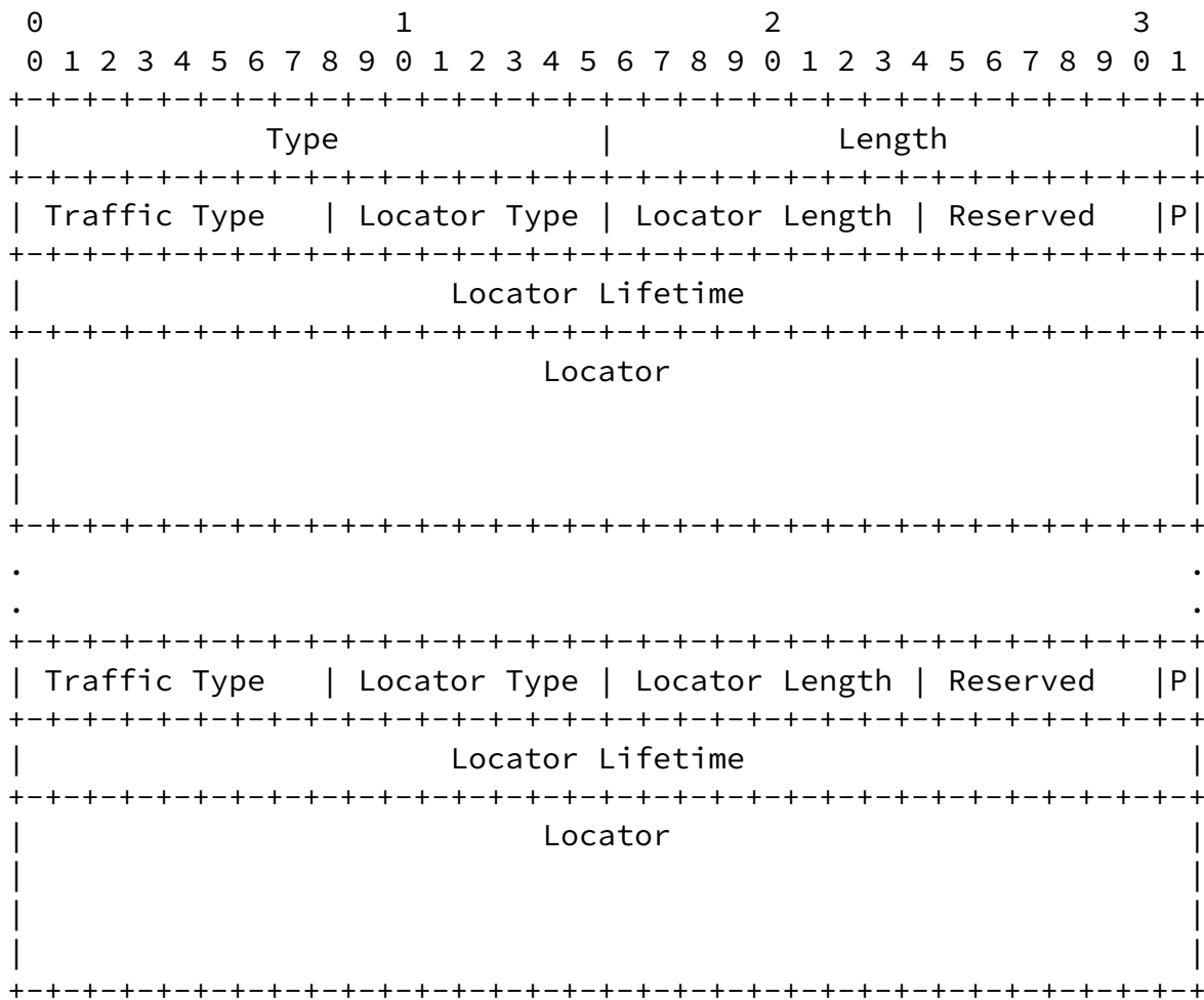
Figure 12: LOCATOR Parameter Format
