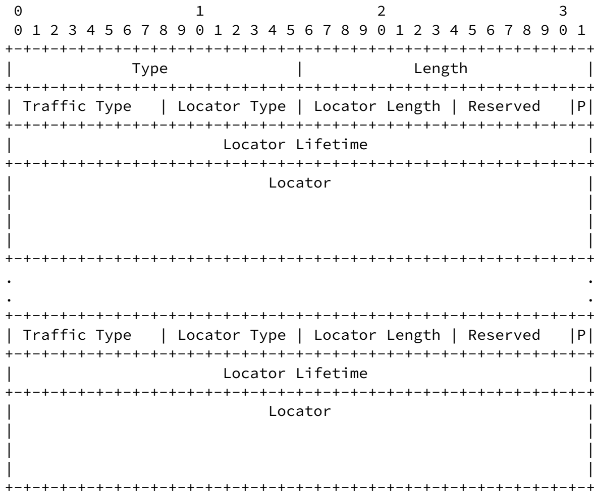
Figure 6: LOCATOR Parameter Format
