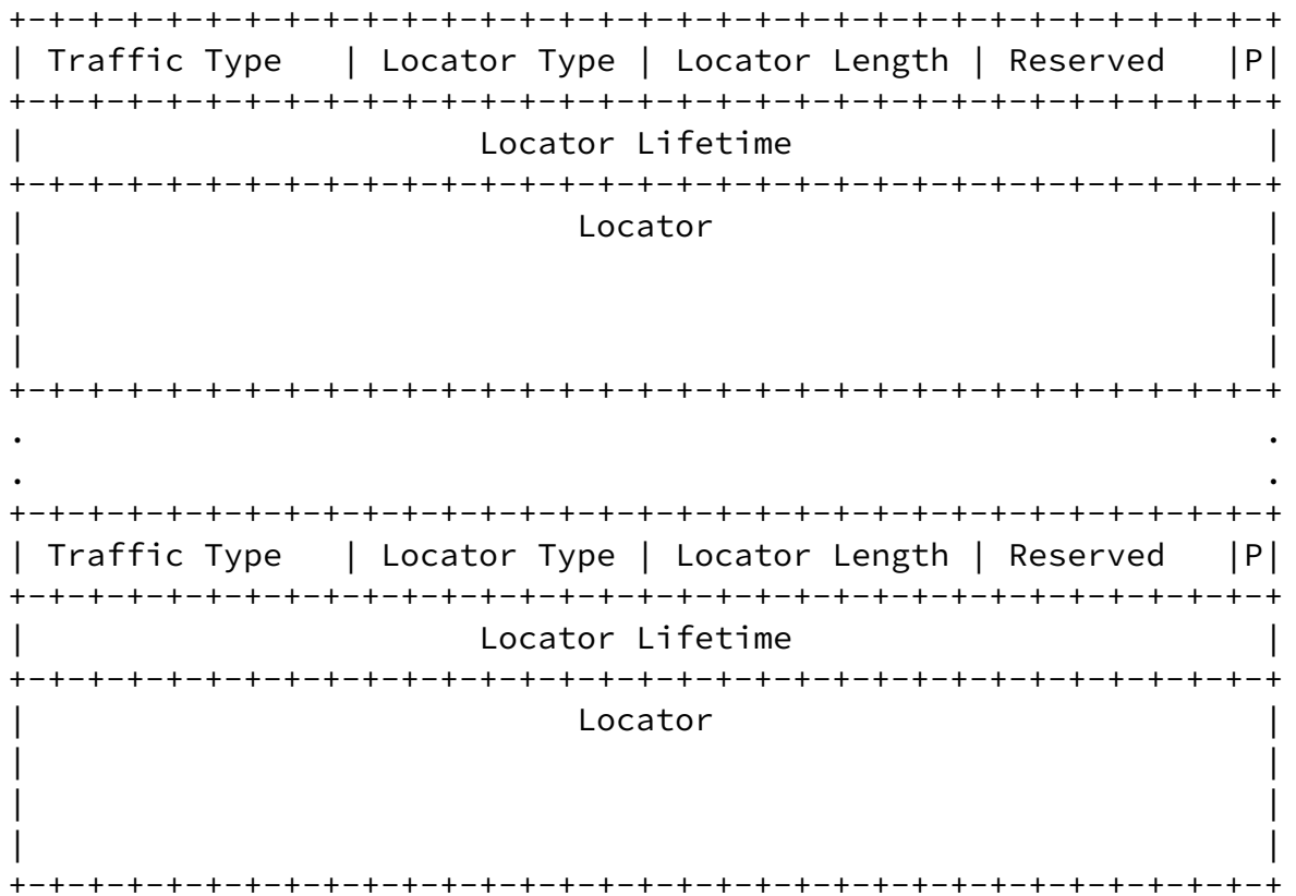
Figure 6: LOCATOR_SET Parameter Format
