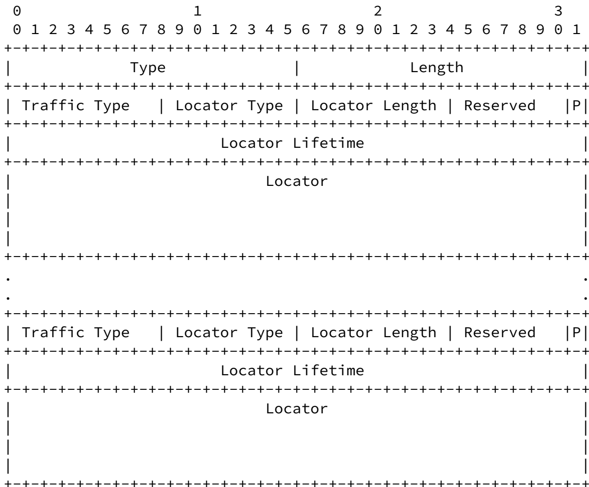
Figure 6: LOCATOR_SET Parameter Format
