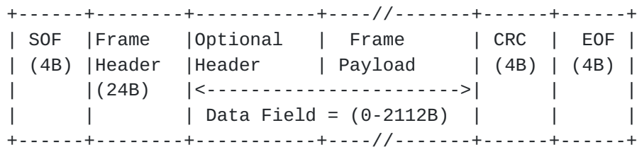
Fig. 1 FC Frame Format
