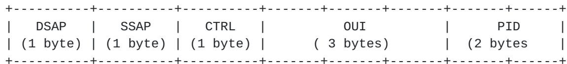
Fig. 8 LLC/SNAP Header
