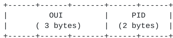
Fig. 7 SNAP Format
