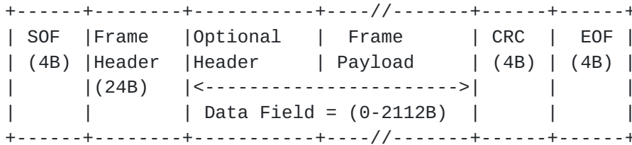
Fig. 16 FC Frame Format
