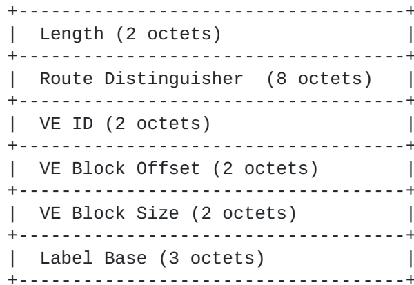
BGP VPLS NLRI
