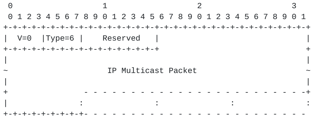
Multicast Data Message Format
