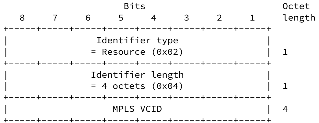
Fig. 4.5: MPLS VCID.
