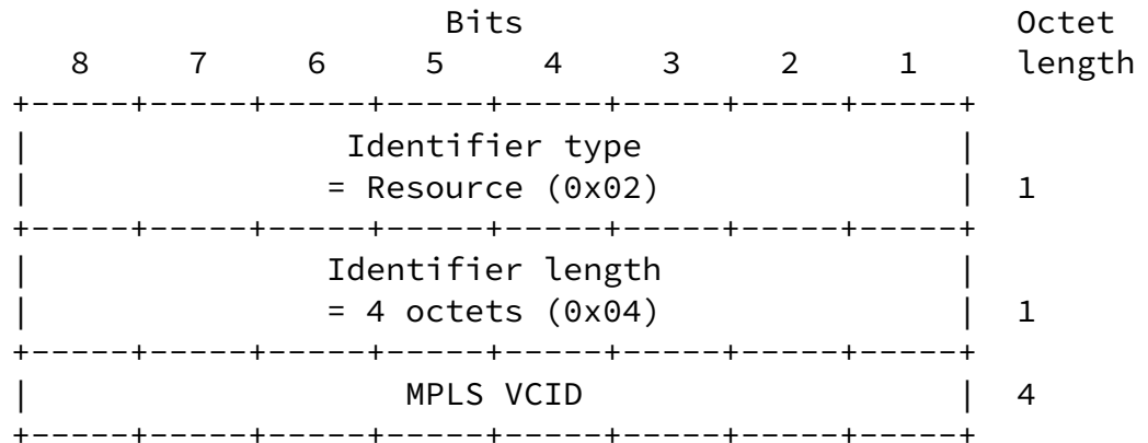
Fig. 4.5: MPLS VCID.
