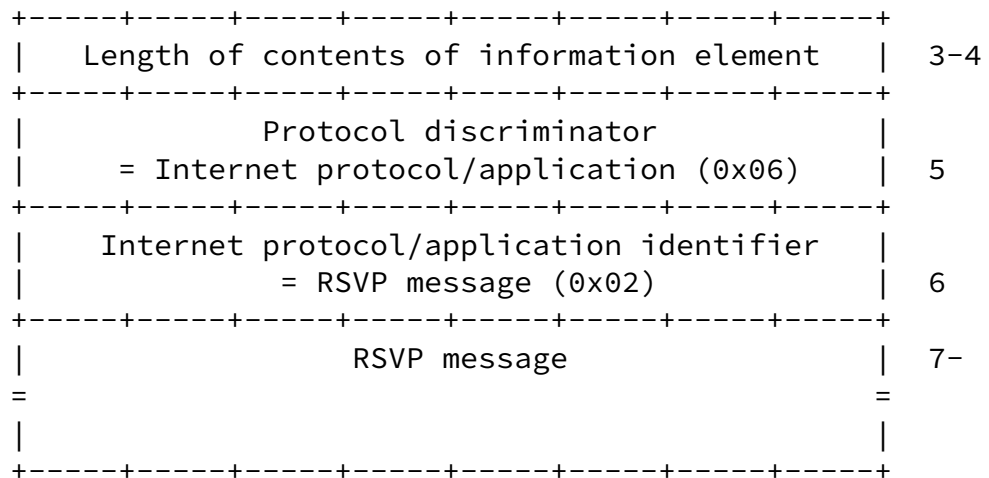
Fig. 4.9: RSVP message.
