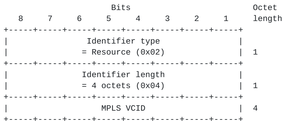
Fig. 4.5: MPLS VCID.
