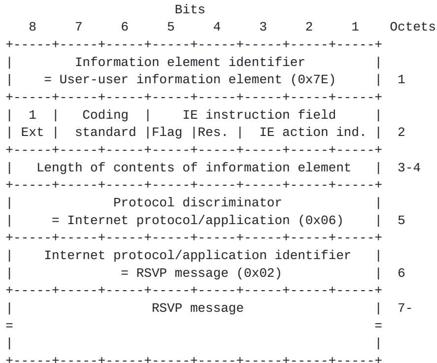
Fig. 4.9: RSVP message.
