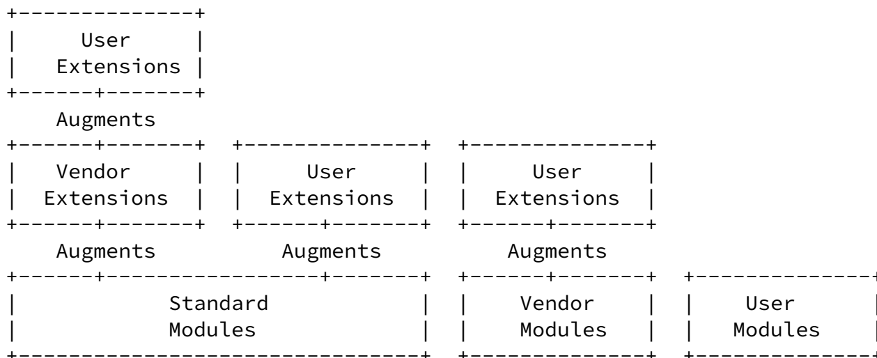
Figure 2: YANG Module Types
