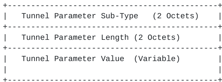
Figure 2: Tunnel Parameter Sub-TLV
