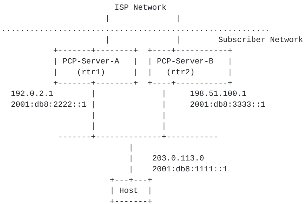
Edge Routers (rtr1, rtr2)
