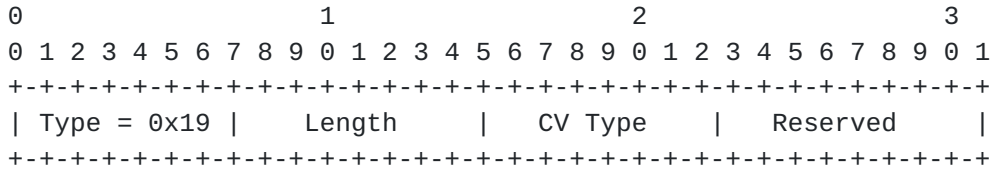
Figure 1: VCCV Extended CV parameter format
