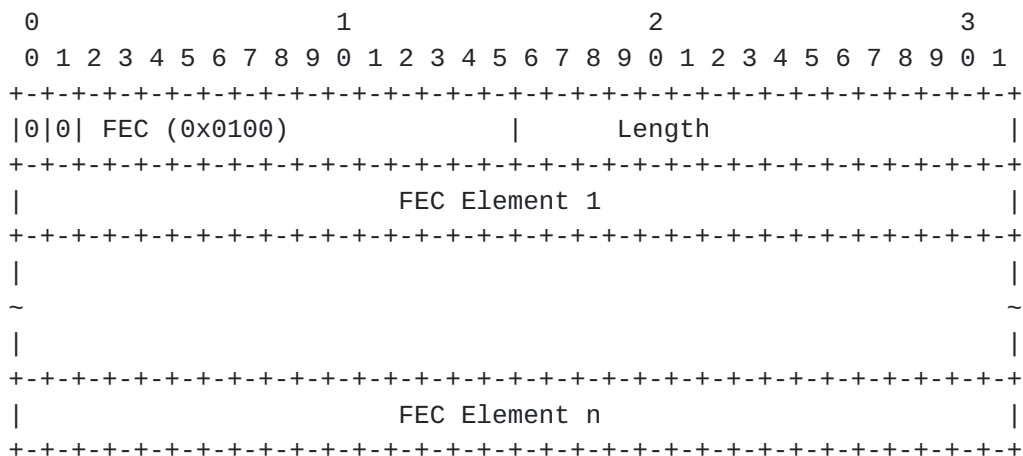
Figure 4: FEC TLV Encoding
