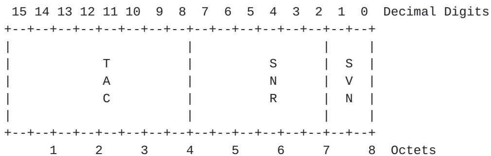
Figure 2. IMEISV Format
