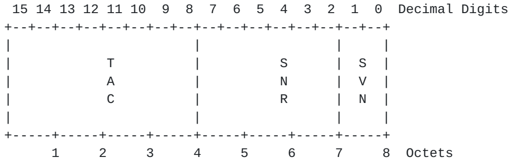
Figure 2. IMEISV Format
