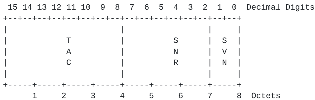
Figure 2. IMEISV Format
