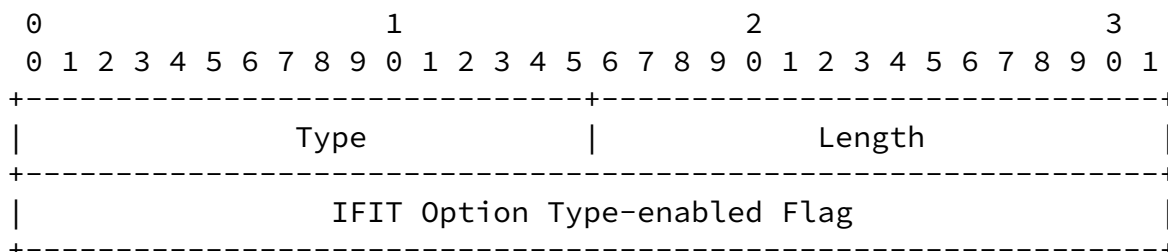
Fig. 1 IFIT Node Capability sub-TLV Format
