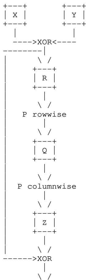
Argon2 compression function G.
